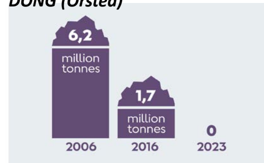
Выбросы CO2 на DONG (Orsted)
